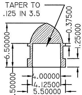
CAP SECTION SCALE: 1.5" = 1.0'
